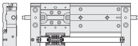
◀ 內部結構圖
